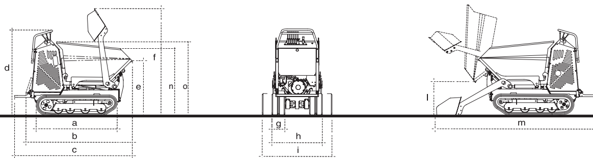
MITAT(mm)
